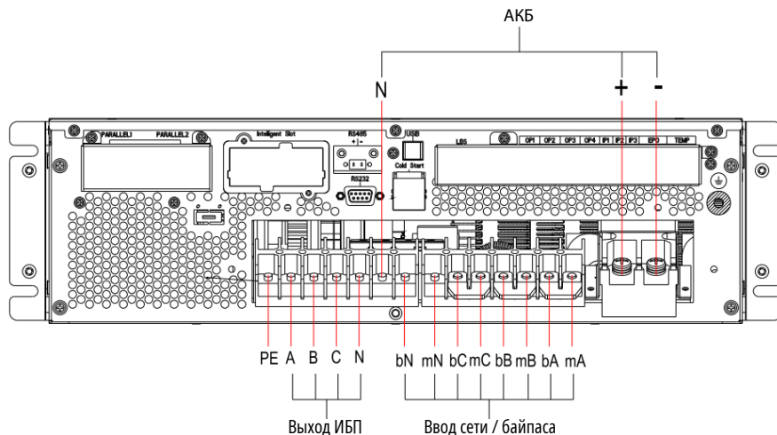
Рисунок 3.15. 3-фазный ввод, 3-фазный выход, общий ввод сети и байпаса
