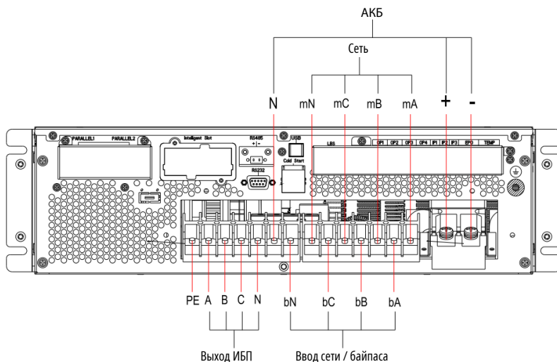
Рисунок 3.16. 3-фазный ввод, 3-фазный выход, отдельный ввод сети и байпаса
