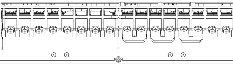
(а) ИБП мощностью 10-30 кВА
