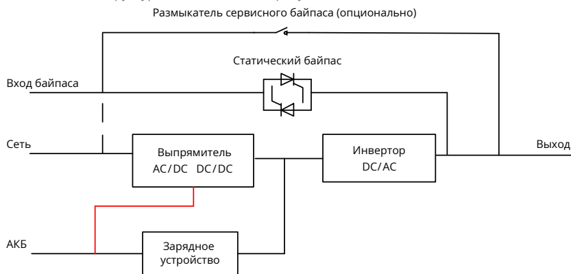
Рисунок 2.3. Структура ИБП
