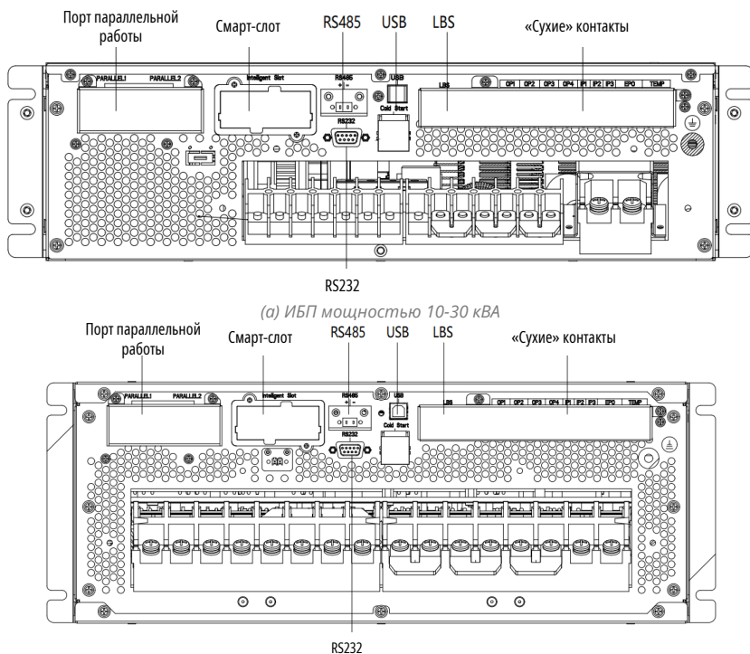
Рисунок 3.7. Коммуникационные интерфейсы и «сухие» контакты
