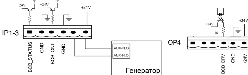
Рисунок 3.11. Порт АВ АКБ
